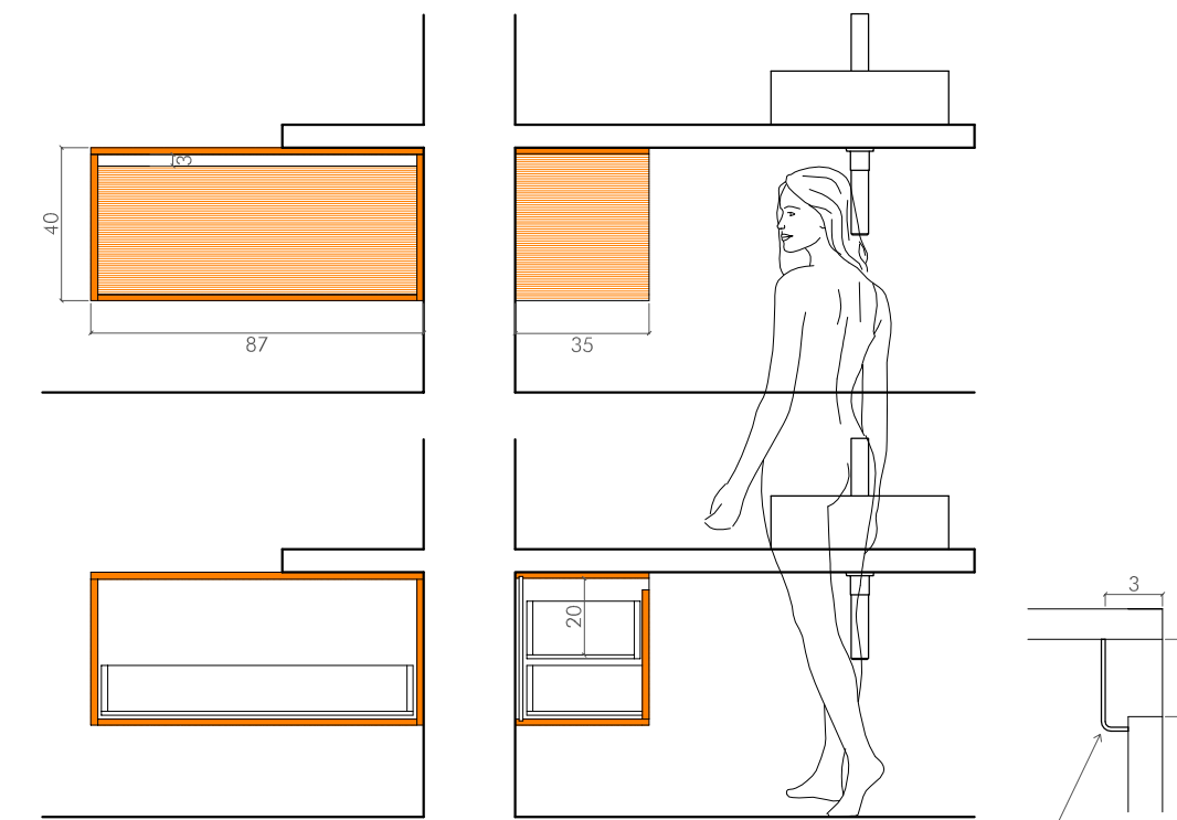
MUEBLE 2 tableros aglomerado 18 mm con chapa en formica naranja. interiores de cajones metal gris. traseros de 10 mm. gola de aluminio suministrada con dos angulos.
