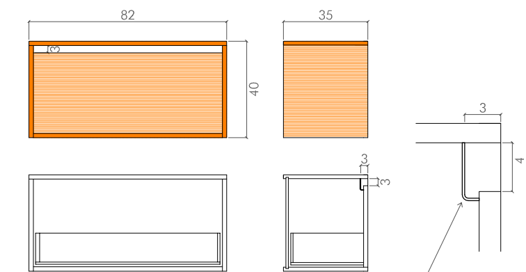
MUEBLE 2 tableros aglomerado 18 mm con chapa en formica naranja. interiores de cajones metal gris. traseros de 10 mm. gola de aluminio suministrada con dos angulos.
